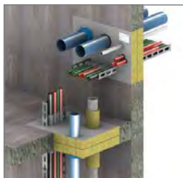
Tesnenie prestupov k blov
